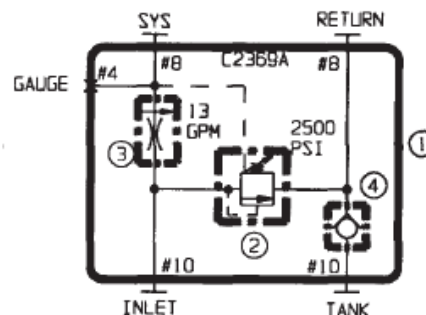
Гидравлическая схема
